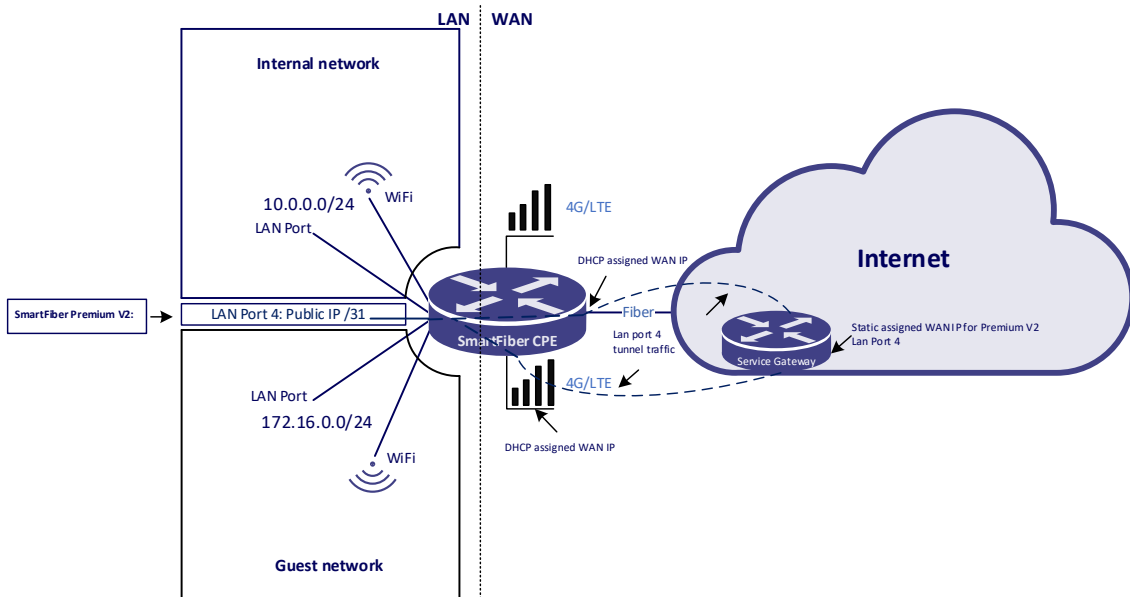
Figur 3: SmartFiber Premium V2
